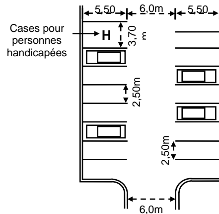
STATIONNEMENT À 90°
