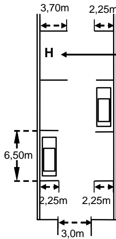
STATIONNEMENT PARALLÈLE
