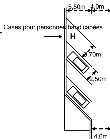
STATIONNEMENT À 30°
